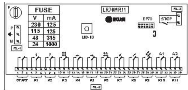
>>> Diagrama bloques salidas receptor
